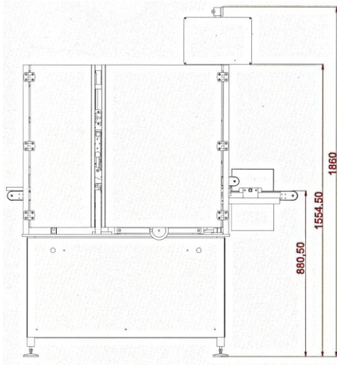
ALZADO DE LA ETIQUETADORA
