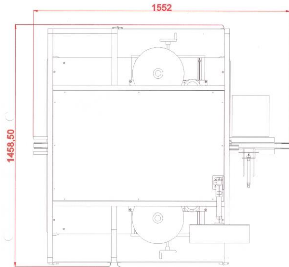
PLANTA DE LA ETIQUETADORA
